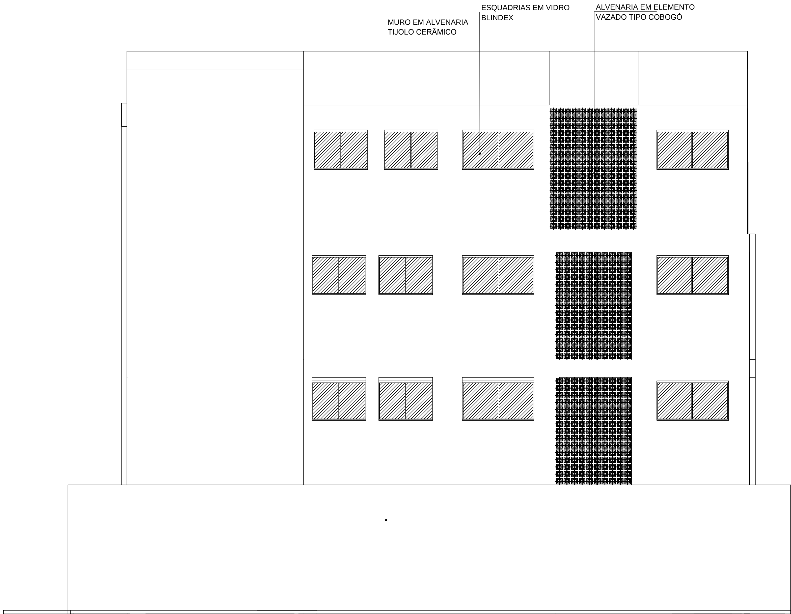
FACHADA LATERAL DIREITA Escala: 1/50
